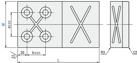
CS30F (Steel type) CS30FN (Steel type without oil groove)
